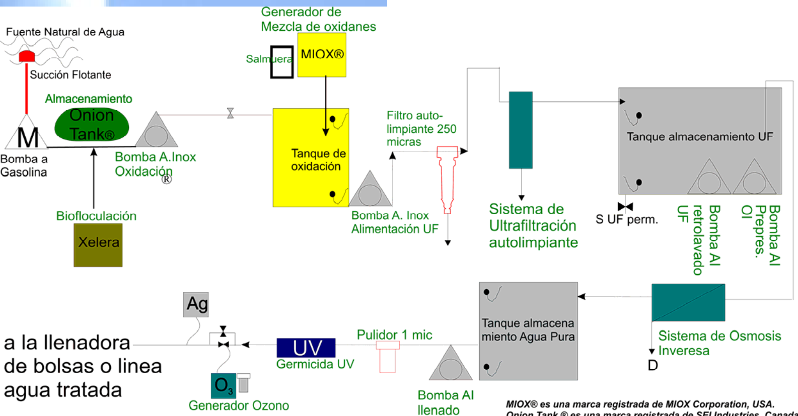
El remolque Portaqua EPS-FirstDrop produce 40,000 litros al día de agua purificada Controlado por el sistema AquaFlex® de Portaqua
